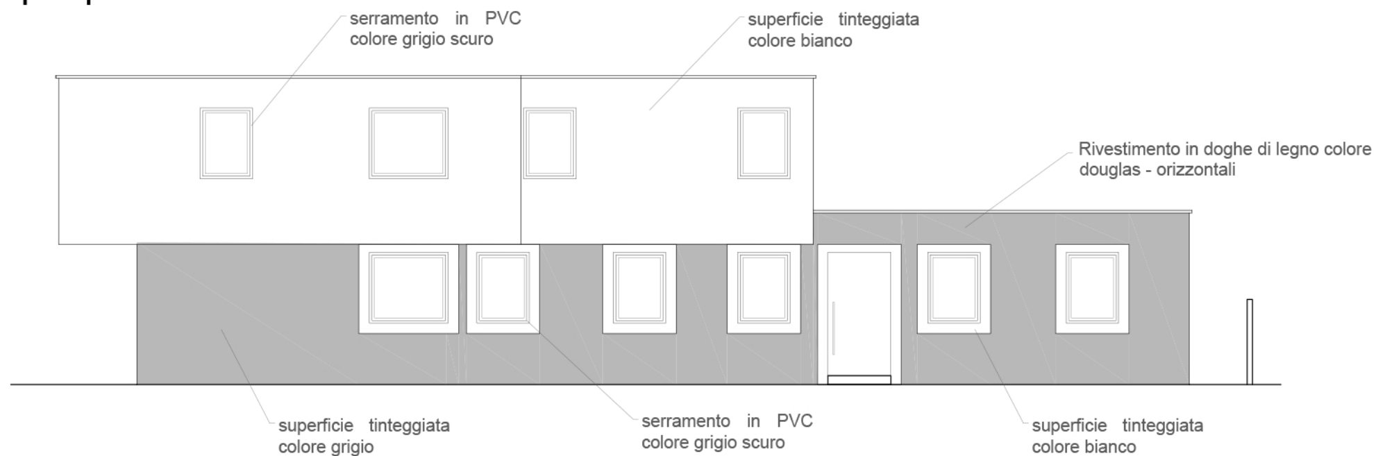
Prospetto Sud - Facciata principale
