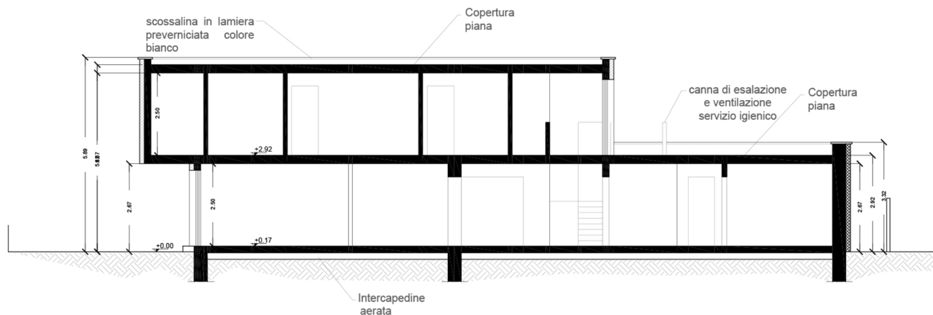
Sezione A-A
