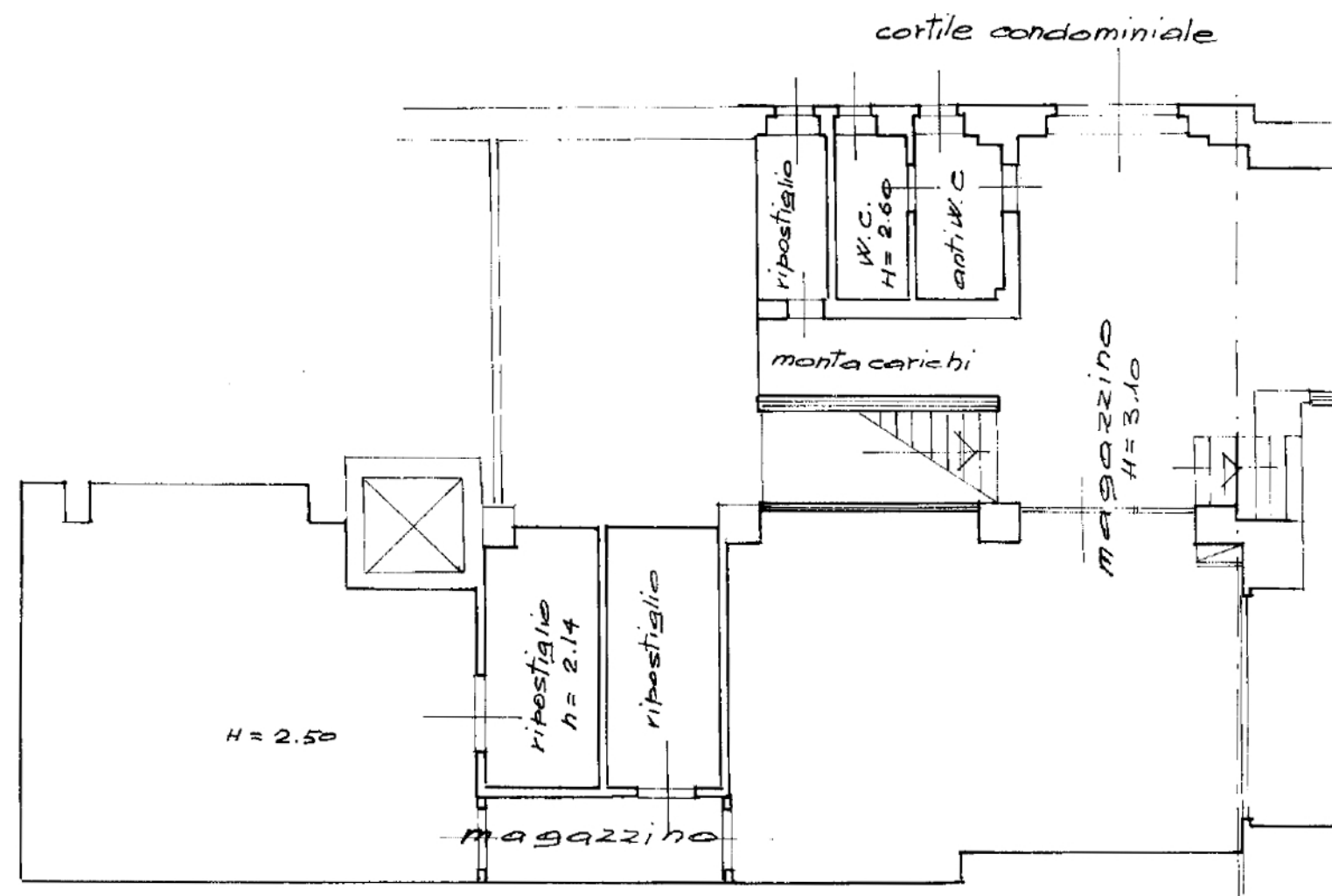
pianta 1° sottoterra
