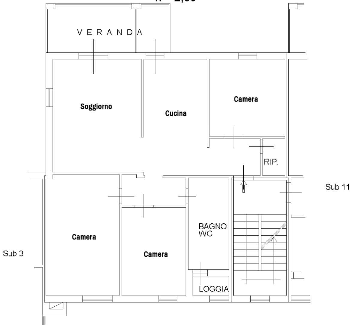
PIANTA PRIMO PIANO h = 2,80
