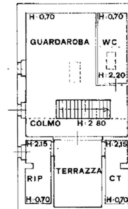
SECONDO PIANO MANSARDATO
