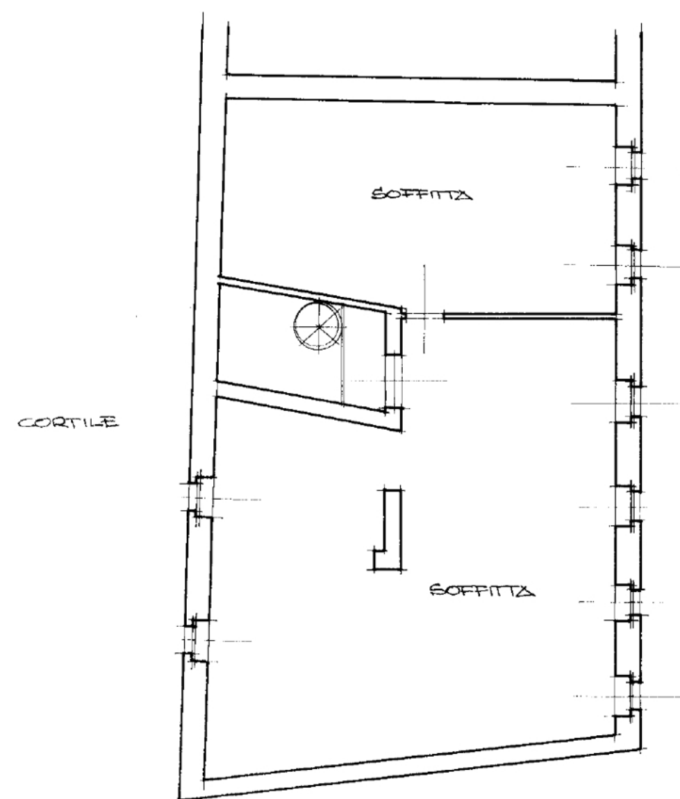
SECONDO PIANO (H = 2.60 - 1.10)
